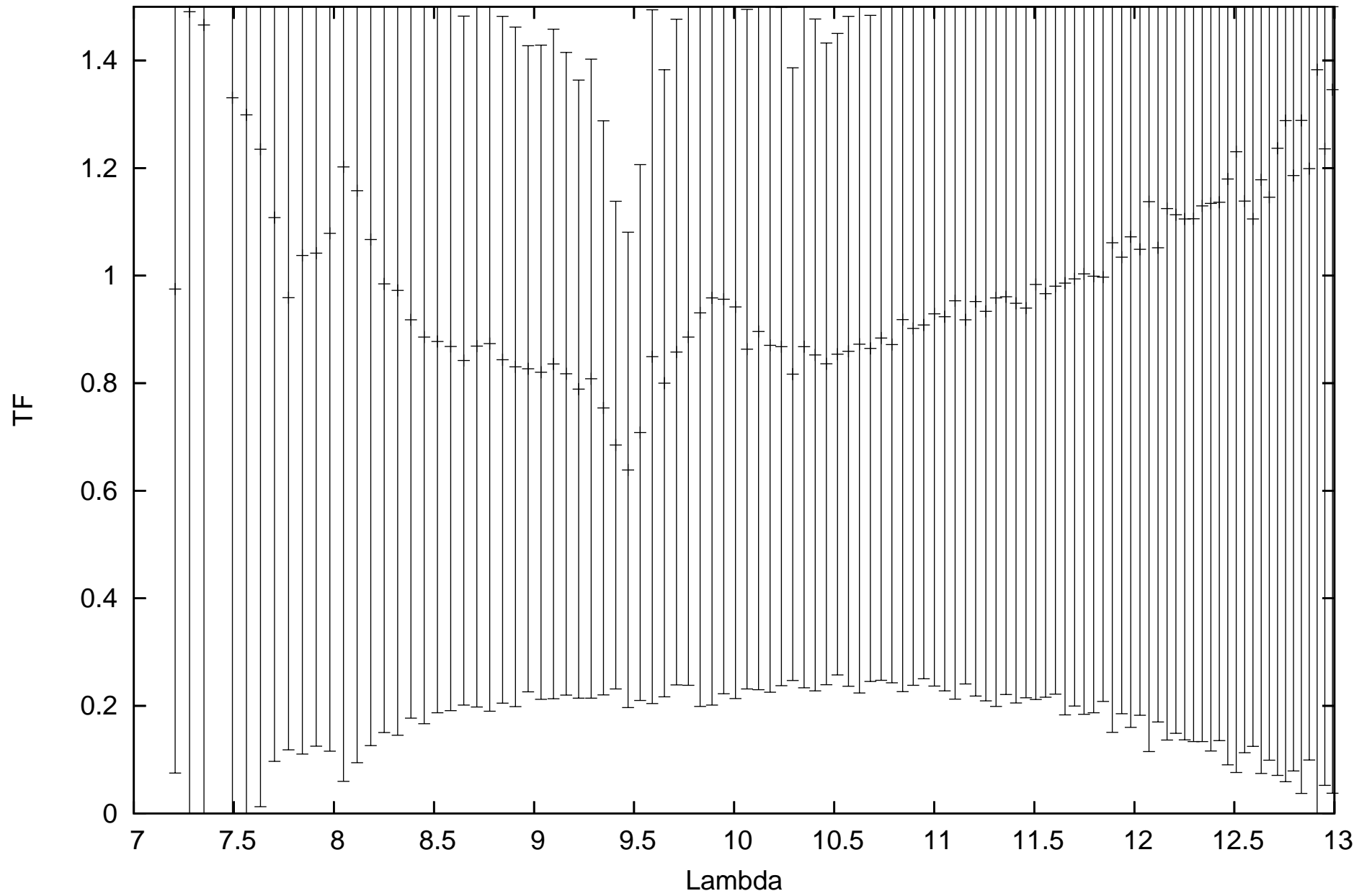
calhd167618_flux-9.9E+100_diam11.86_r.MIDI.2008-10-01T00_34_31.138 SCIPHOT
