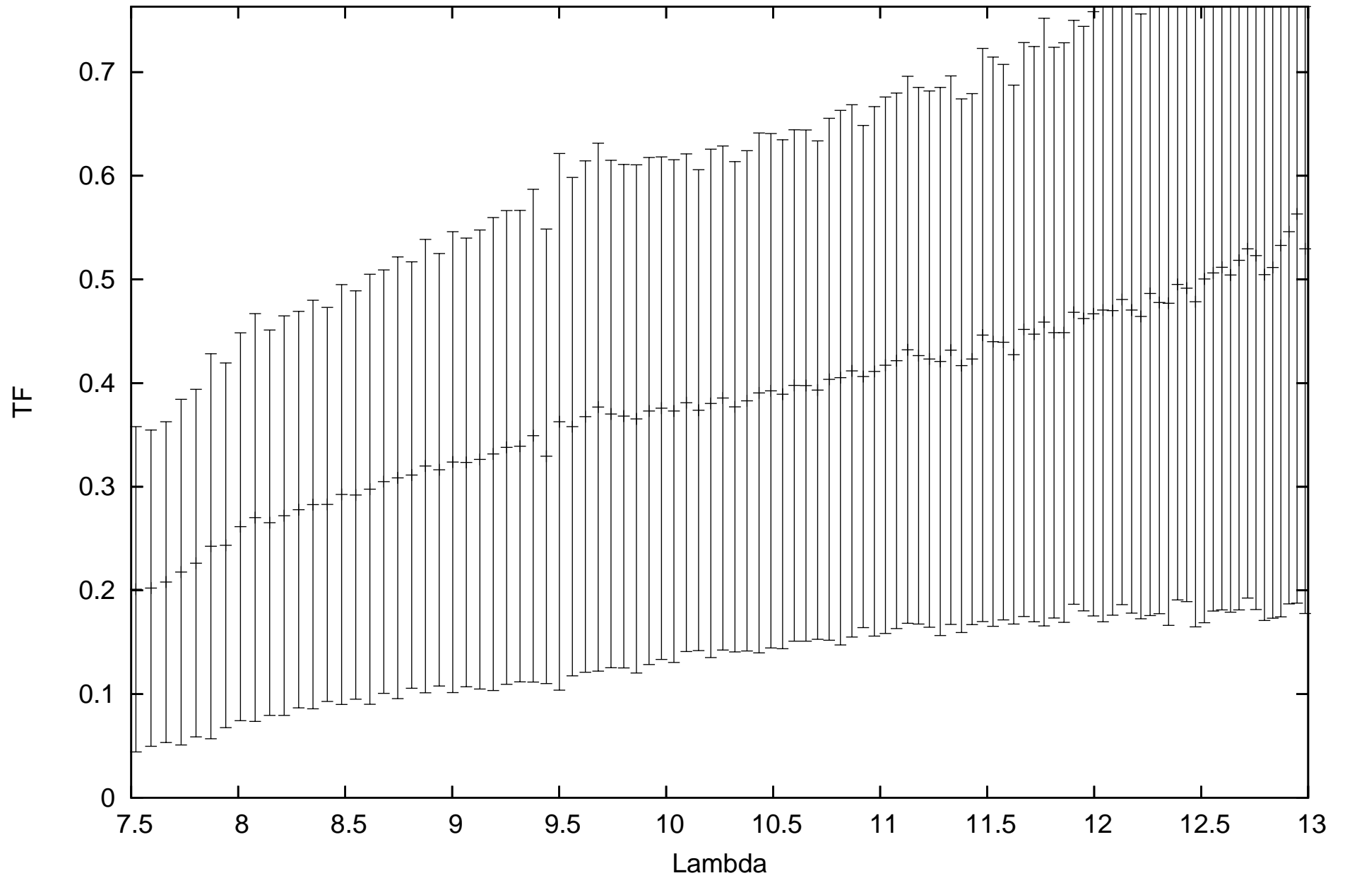
calHD167618_flux-1.82_diam11.66_r.MIDI.2011-06-24T08_50_04.000_G111
