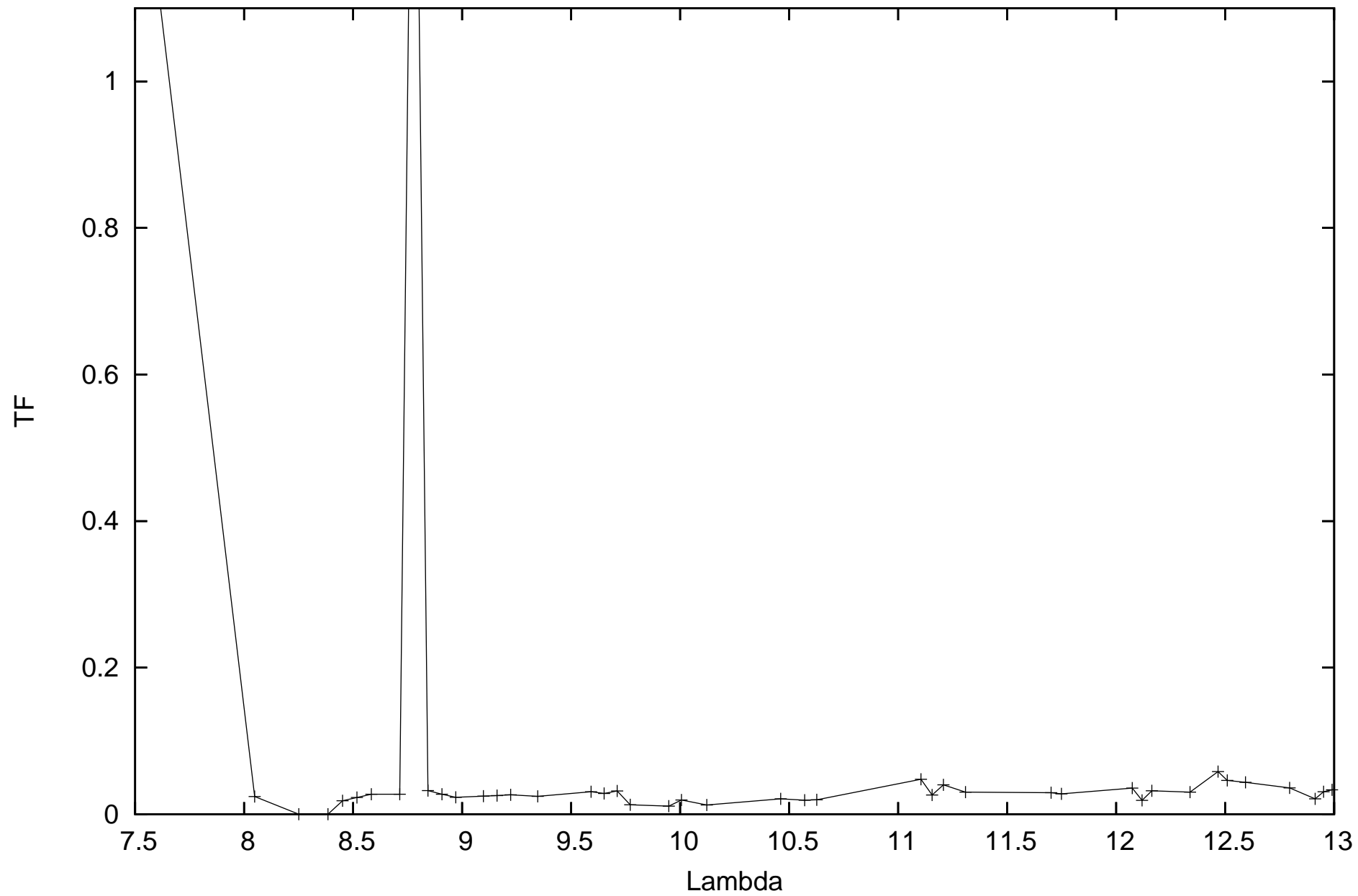
calHD085503_flux1.09_diam2.77_r.MIDI.2011-01-18T06_50_52.973_U2U3
