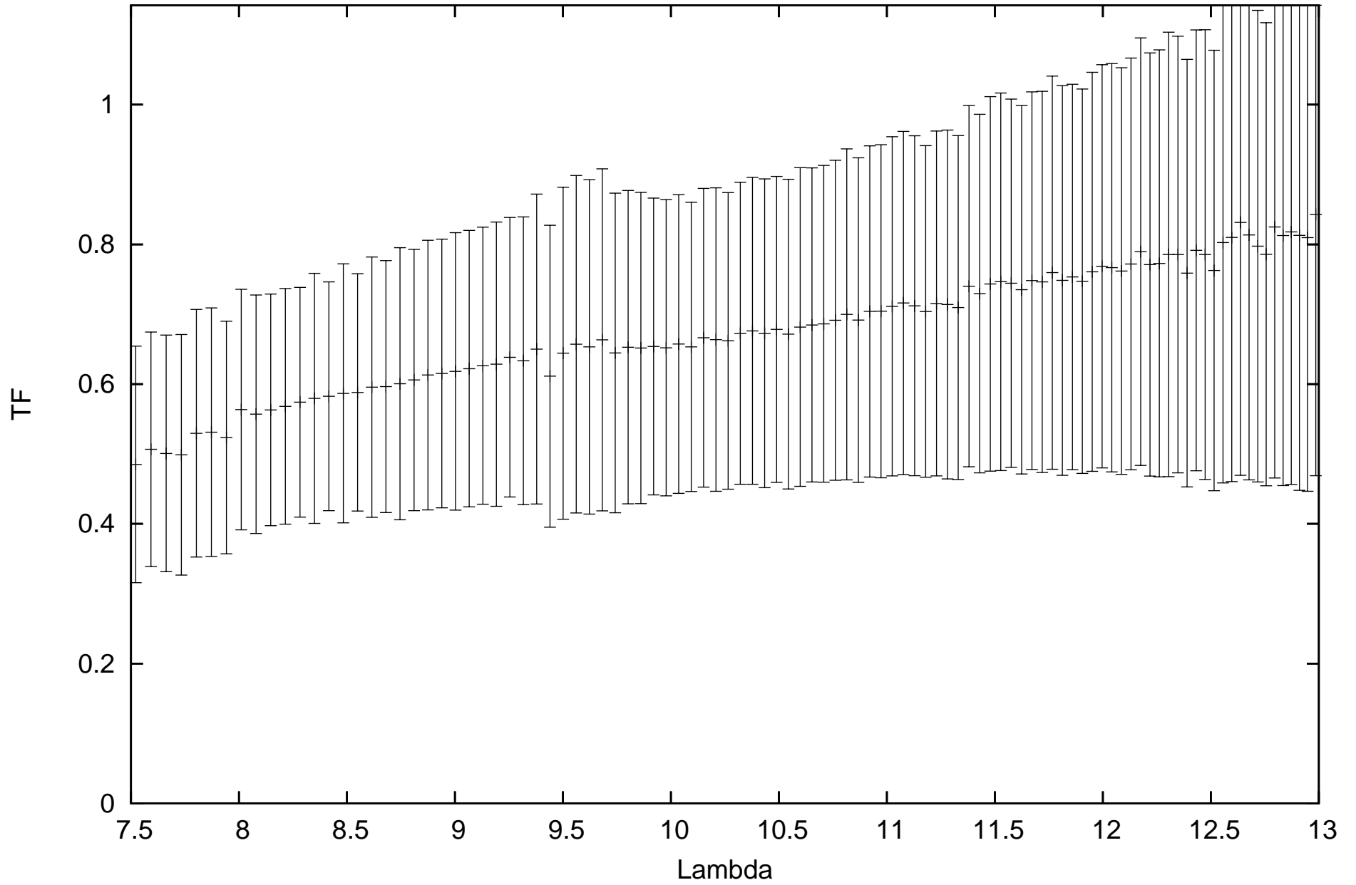
calHD120404_flux1.19_diam2.96_r.MIDI.2011-03-21T04_30_54.000_U3U4
