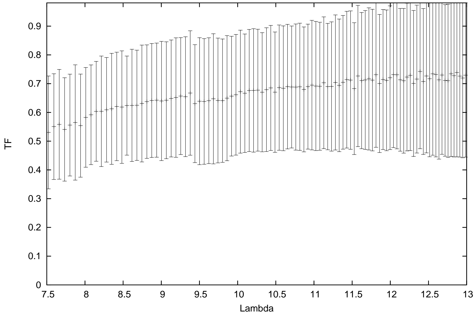
calHD159881_flux1.59_diam2.46_r.MIDI.2011-05-13T09_23_25.000_U3U4
