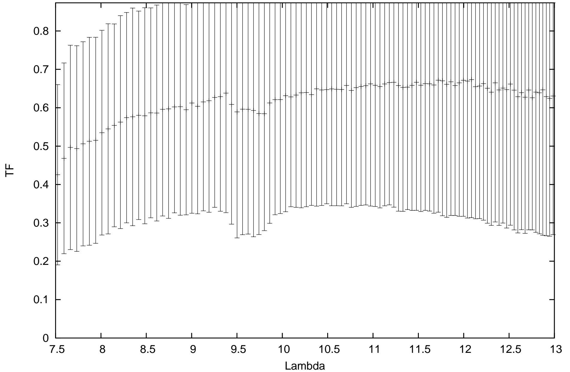
calHD167618_flux-1.82_diam11.66_r.MIDI.2011-09-05T04_52_12.000_G111
