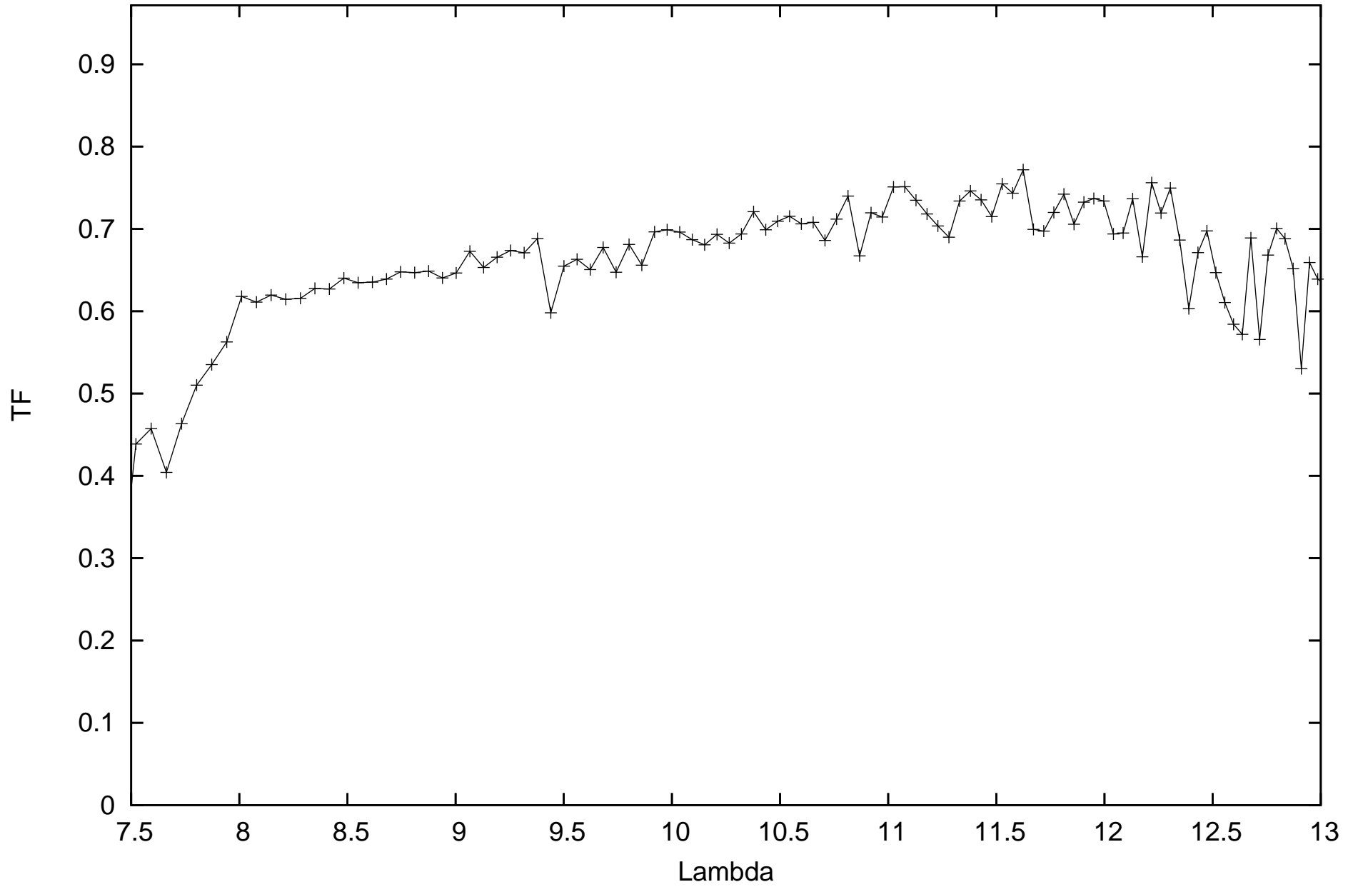
calHIP90739_flux2.96997_diam1.269283_r.MIDI.2011-04-15T06_02_18.000_U2U3
