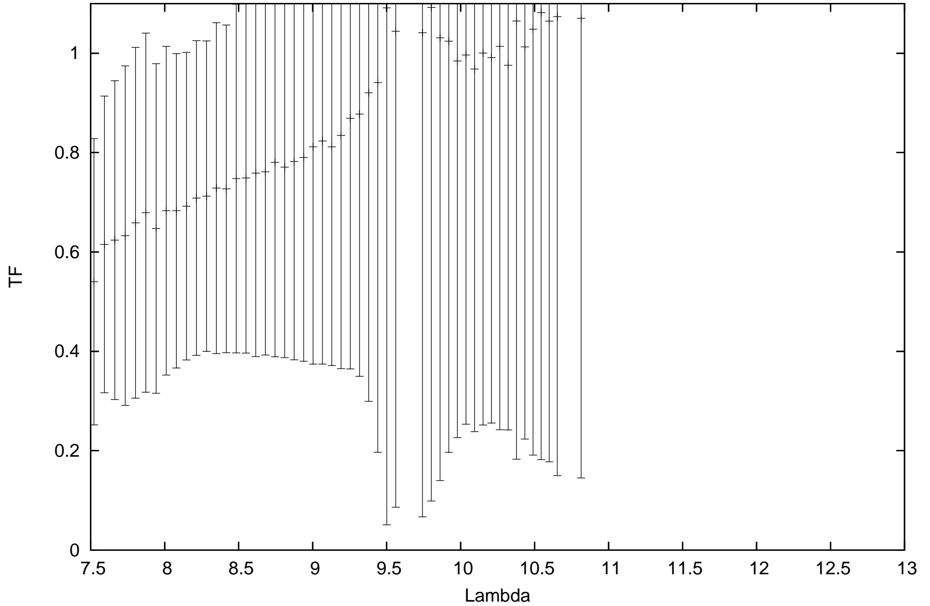
calHIP90739_flux2.96997_diam1.269283_r.MIDI.2011-04-17T07_30_50.000_U3U4
