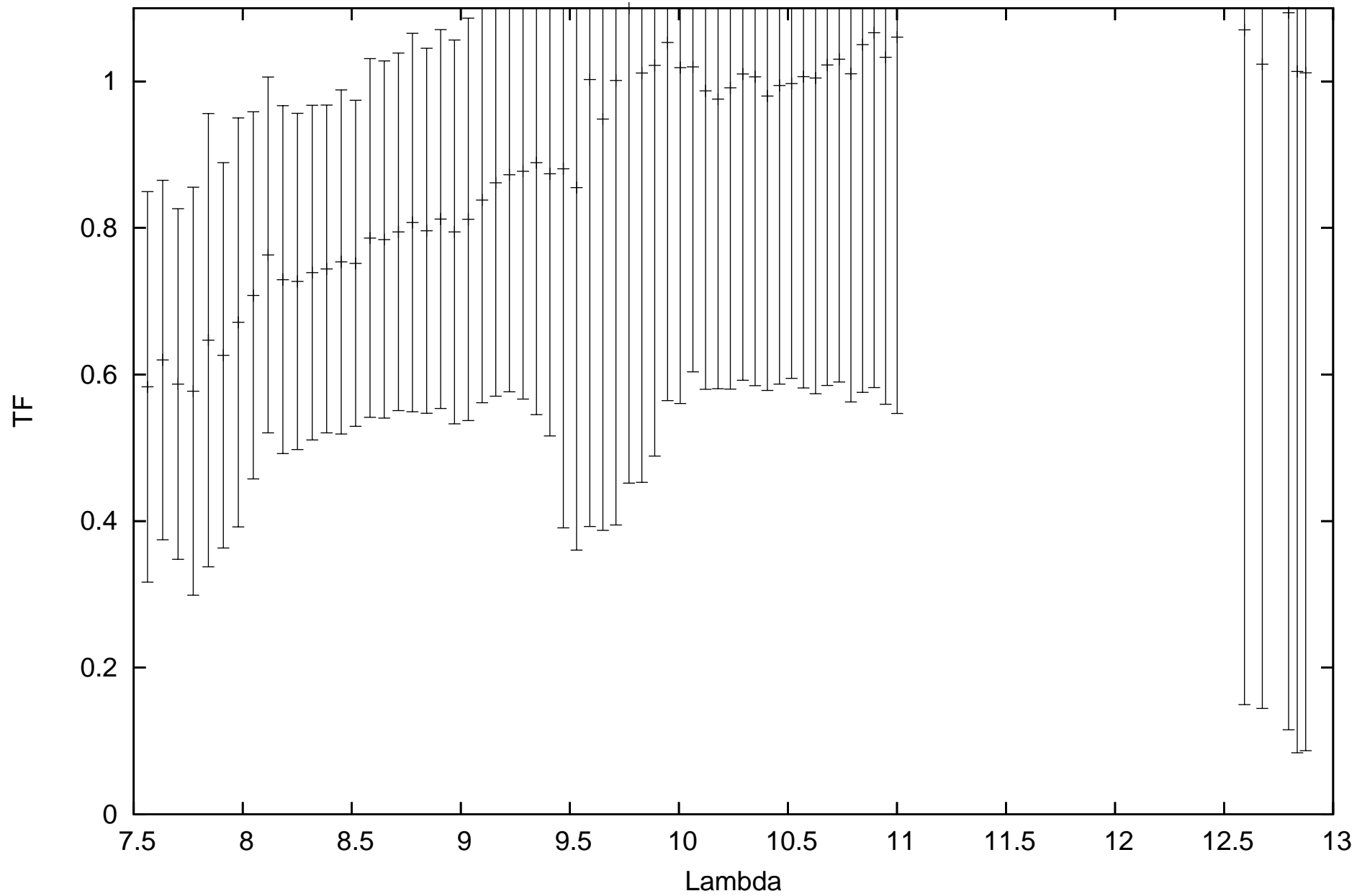
calHD167618_flux-1.82_diam11.66_r.MIDI.2012-09-22T02_50_52.113_C1B2
