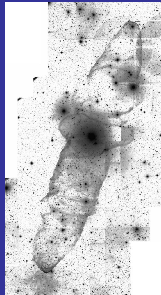
Ou4: Young stellar object (Romano Corradi)
