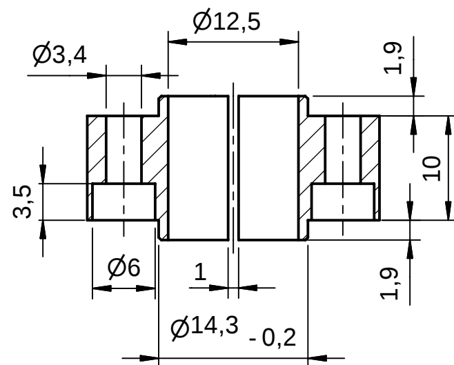
B-B ( 2 : 1 )
