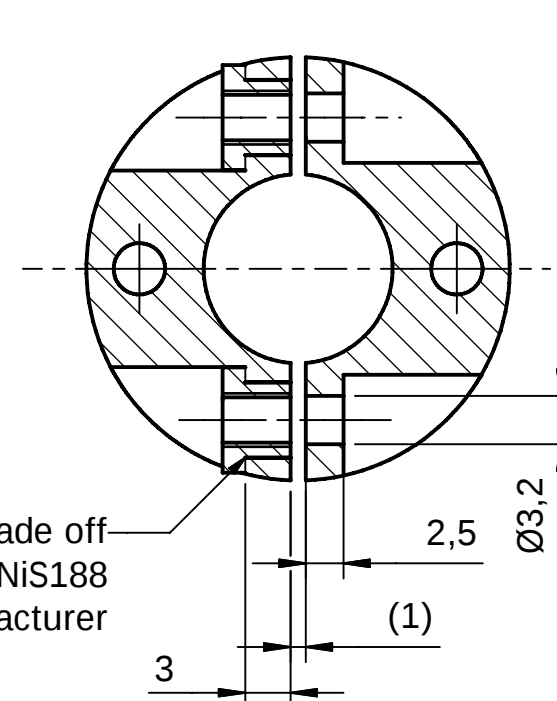
A-A ( 2 : 1 )
