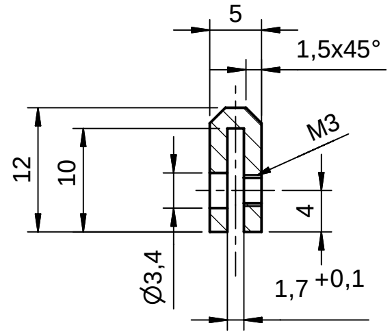
A-A ( 2 : 1 )
