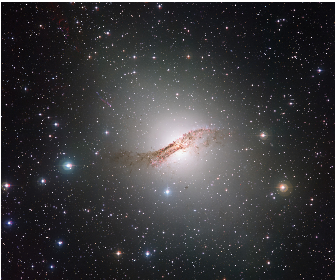
The galaxy Centaurus A (NGC 5128).
