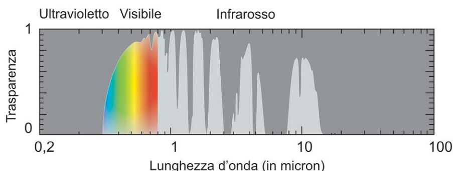
Figura 1: Assorbimento della radiazione da parte dell'atmosfera terrestre
